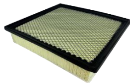
EAM 2271 58 x 270 x 240 17801-31160 AIRE
