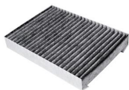
MHC 740 220 x 30 x 156 51979427 HABTACULO CARBON ACTIVADO
