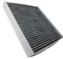
MHC 729 254 x 36 x 222 6R0 819 653 HABITACULO CARBON ACTIVADO
